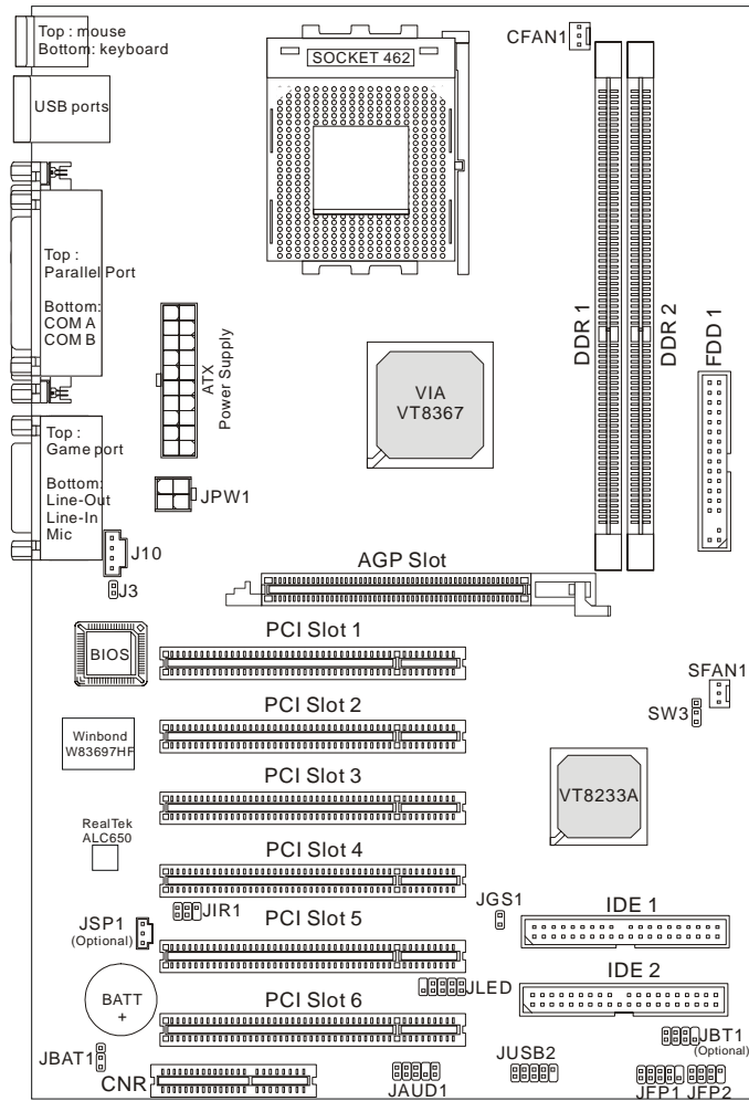
KT3 Ultra-C (MS-6593 v1.X) ATX Mainboard
